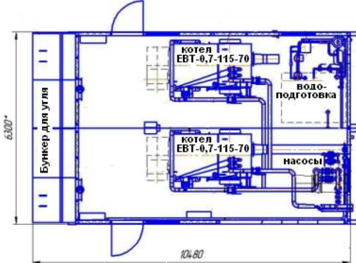
Котельная установка УKM-1,4BP (топливо – уголь) 1,4 МВт; температура воды – 115 °С
